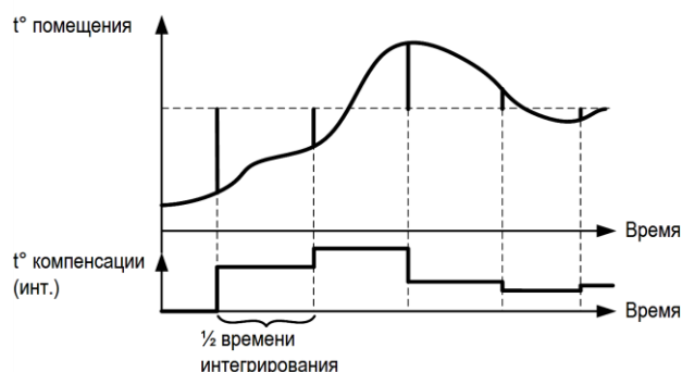
Изменение интегральной составляющей компенсации
