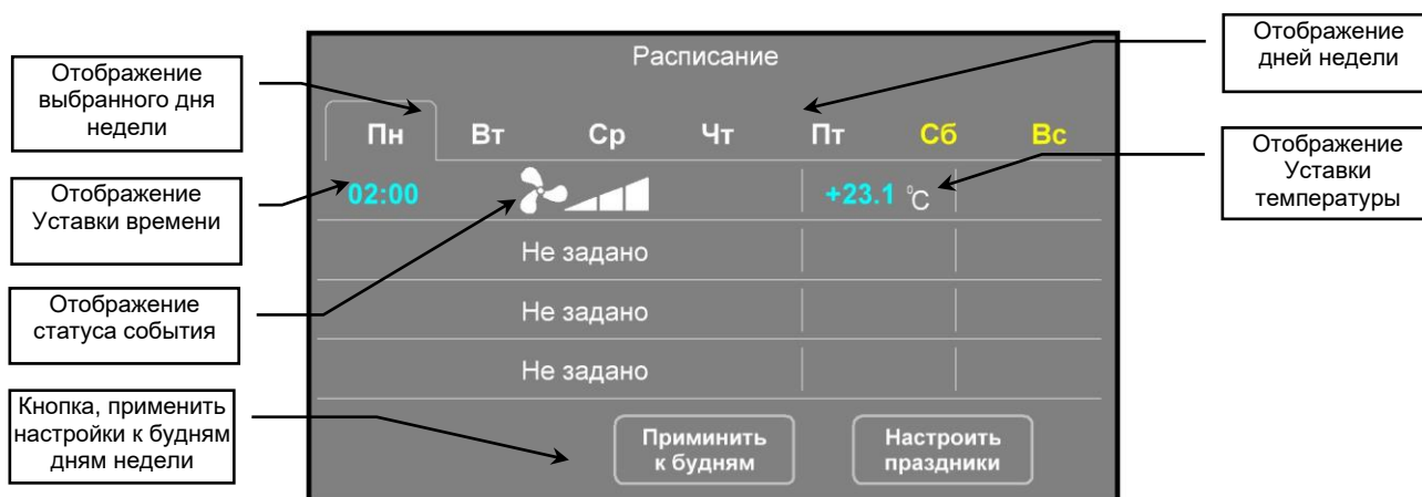
Рисунок 6 - Экран редактирования расписания контроллера SMH4
