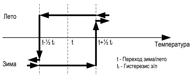
Рисунок 2 – Гистерезис перехода «зима»-«лето»
