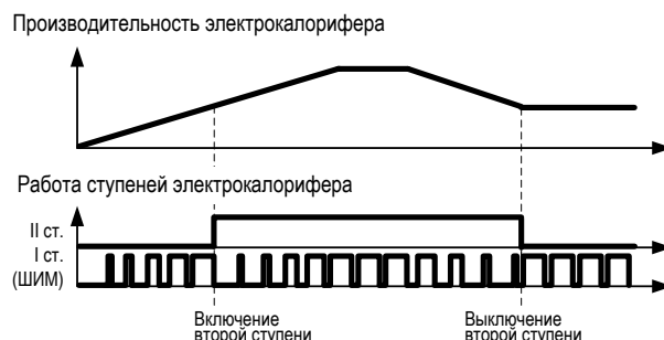
Рисунок 13 – Диаграмма работы электрического нагревателя
