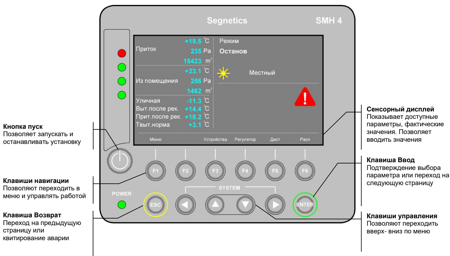
Рисунок 2 - Общий вид управляющего контроллера SMH4
