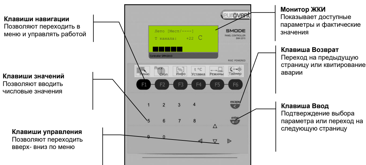
Рисунок 1 - Общий вид управляющего контроллера SMH2010
