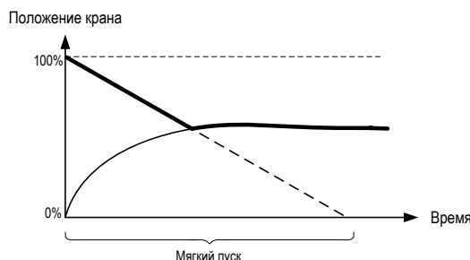
Рисунок 11 - Мягкий пуск. Метод «2»
