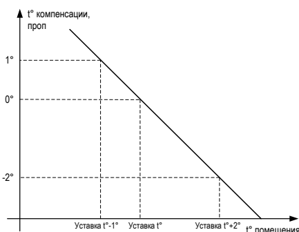
Рисунок 15 – Пример вычисления пропорциональной составляющей уставки
